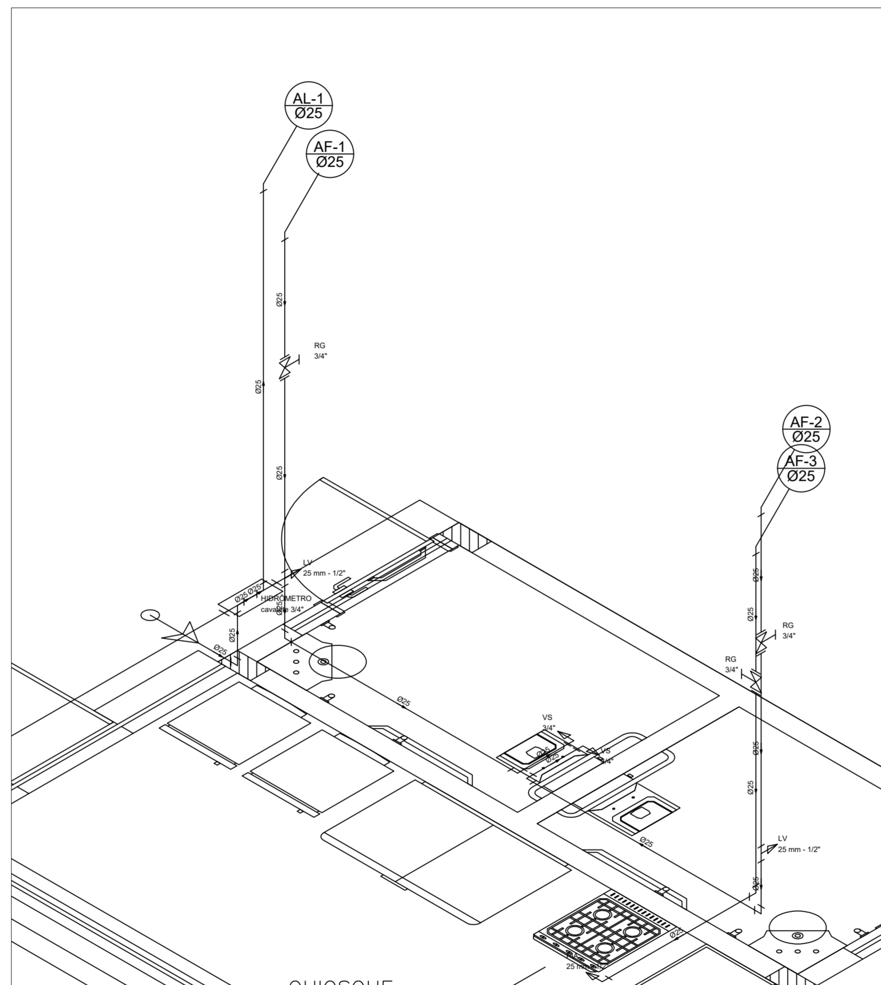
DETALHE 02 Campos, Maxaranguape/RN 1/20
