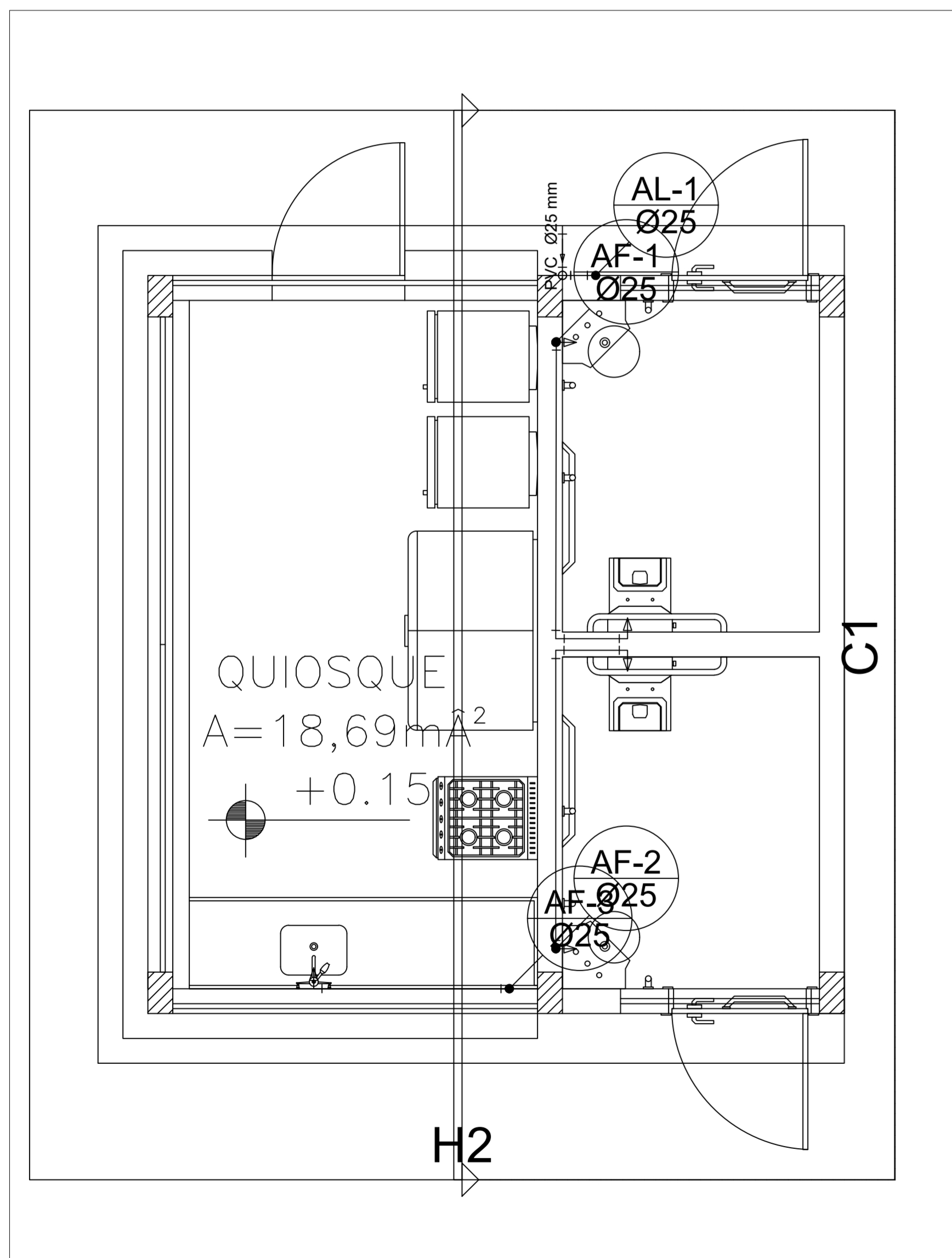
PLANTA DE SITUAÇÃO Campos, Maxaranguape/RN Sem escala
